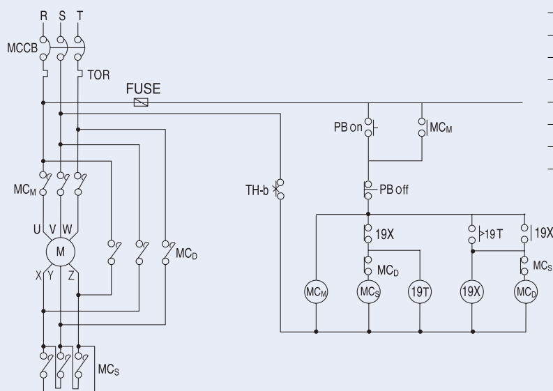
(Рис. 1) Пример схемы подключения с переключением звезда-треугольник
